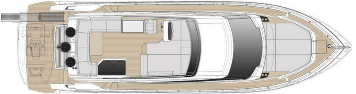
Flybridge
